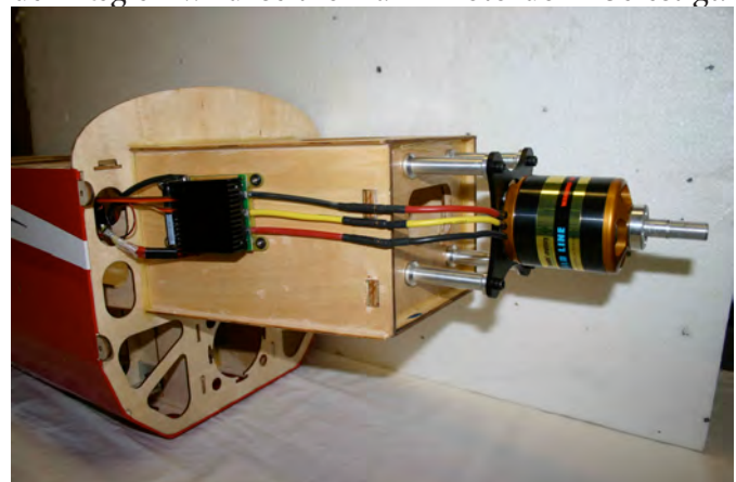
Abbildung 29: AXI 5345, Jeti Spin pro 125
