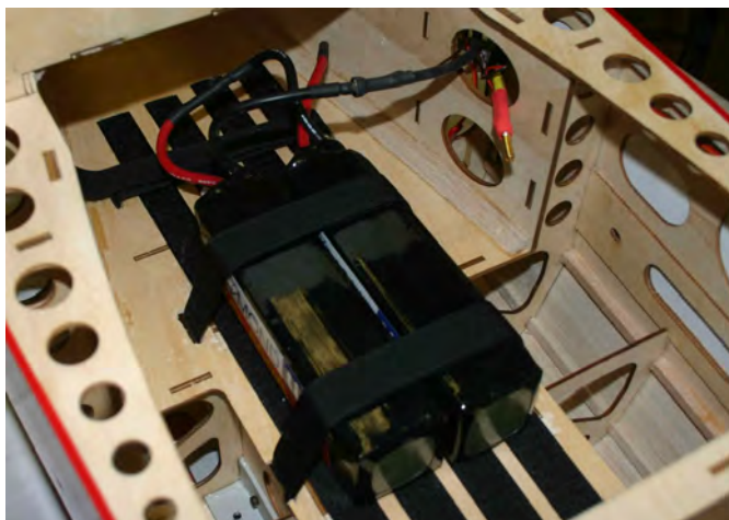
Abbildung 41: Antriebsakku
