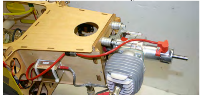
Abbildung 34: DA-60, Zündung und Gasservo
